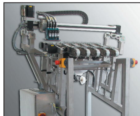
Маркировочная установка
