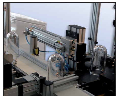
Маркировка сосудов
