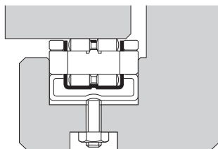
(а) Использование специального ограничителя
