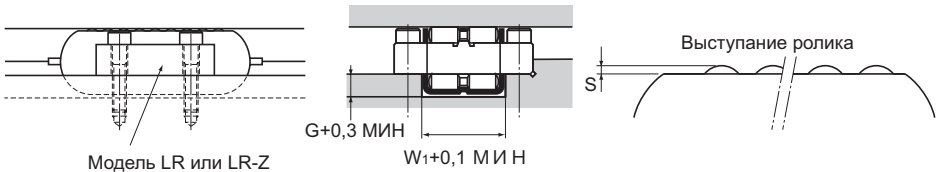
Модель LR или LR-Z
